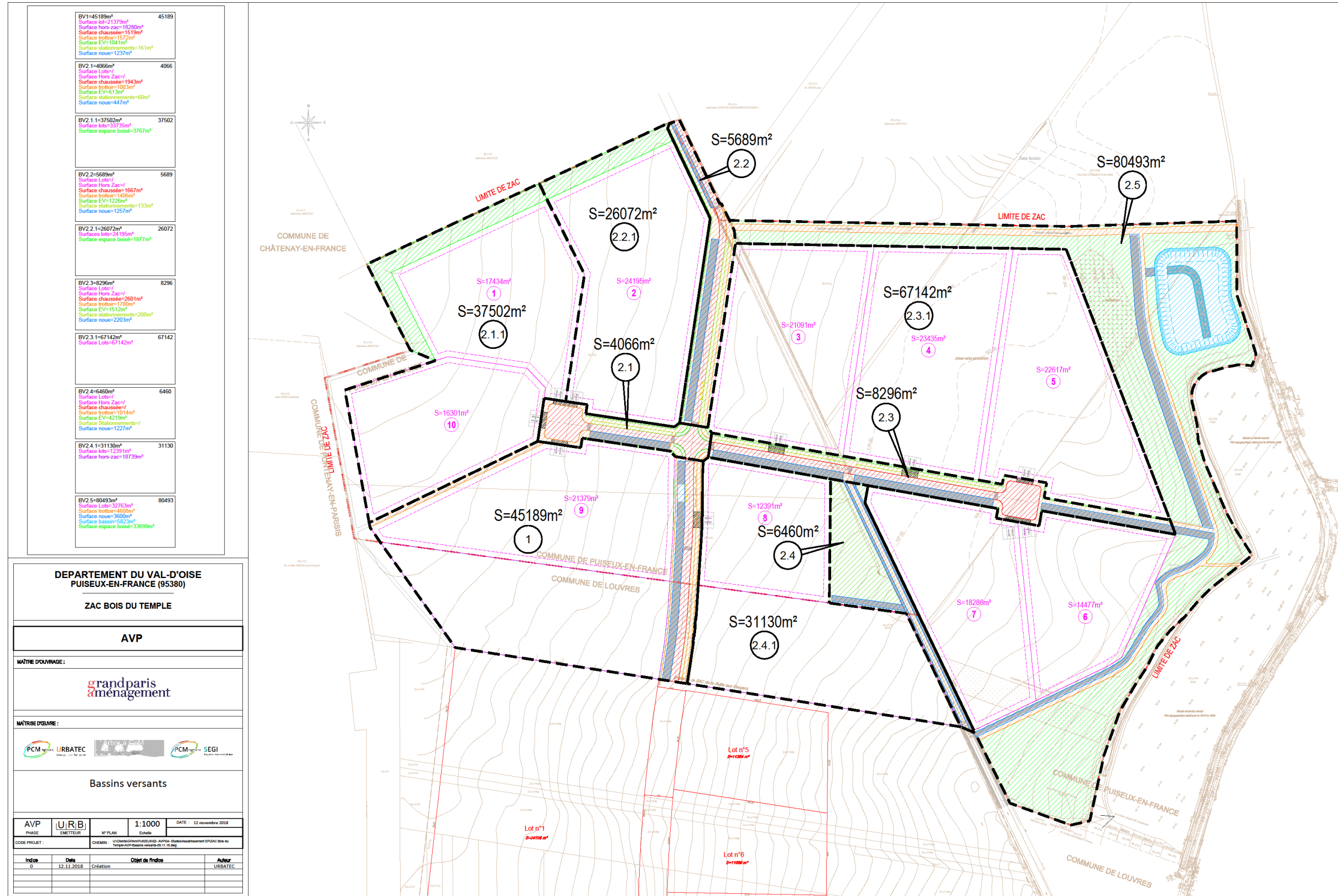
Figure 44 : Bassins versants hydrologiques de la ZA
