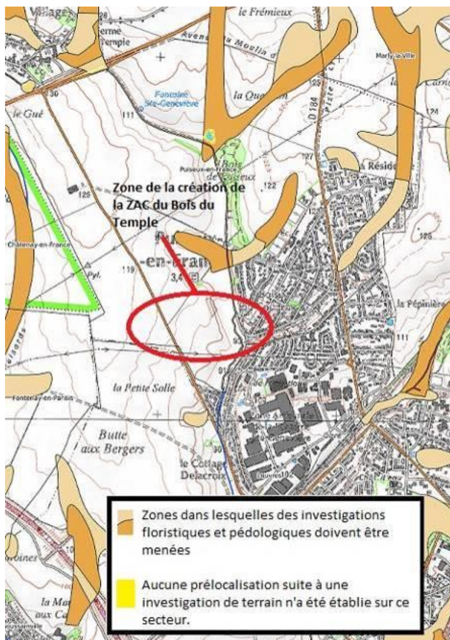
Figure 21 : Carte des zones humides du secteur affinée par le SAGE CEVM
