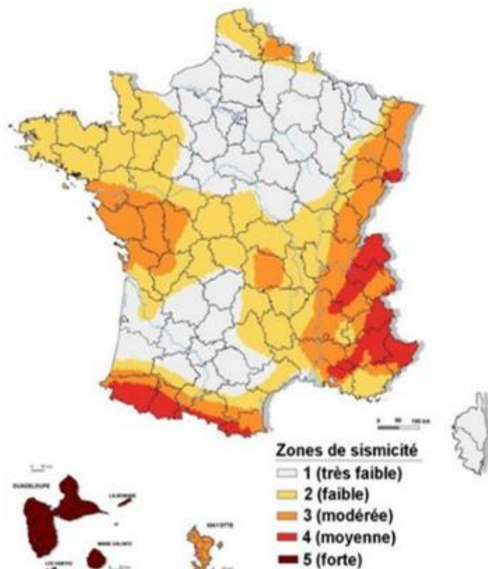
Figure 26 : Nouveau zonage sismique en France
