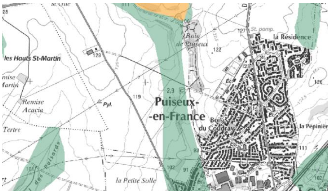
Figure 20 : Cartes des zones humides du secteur
