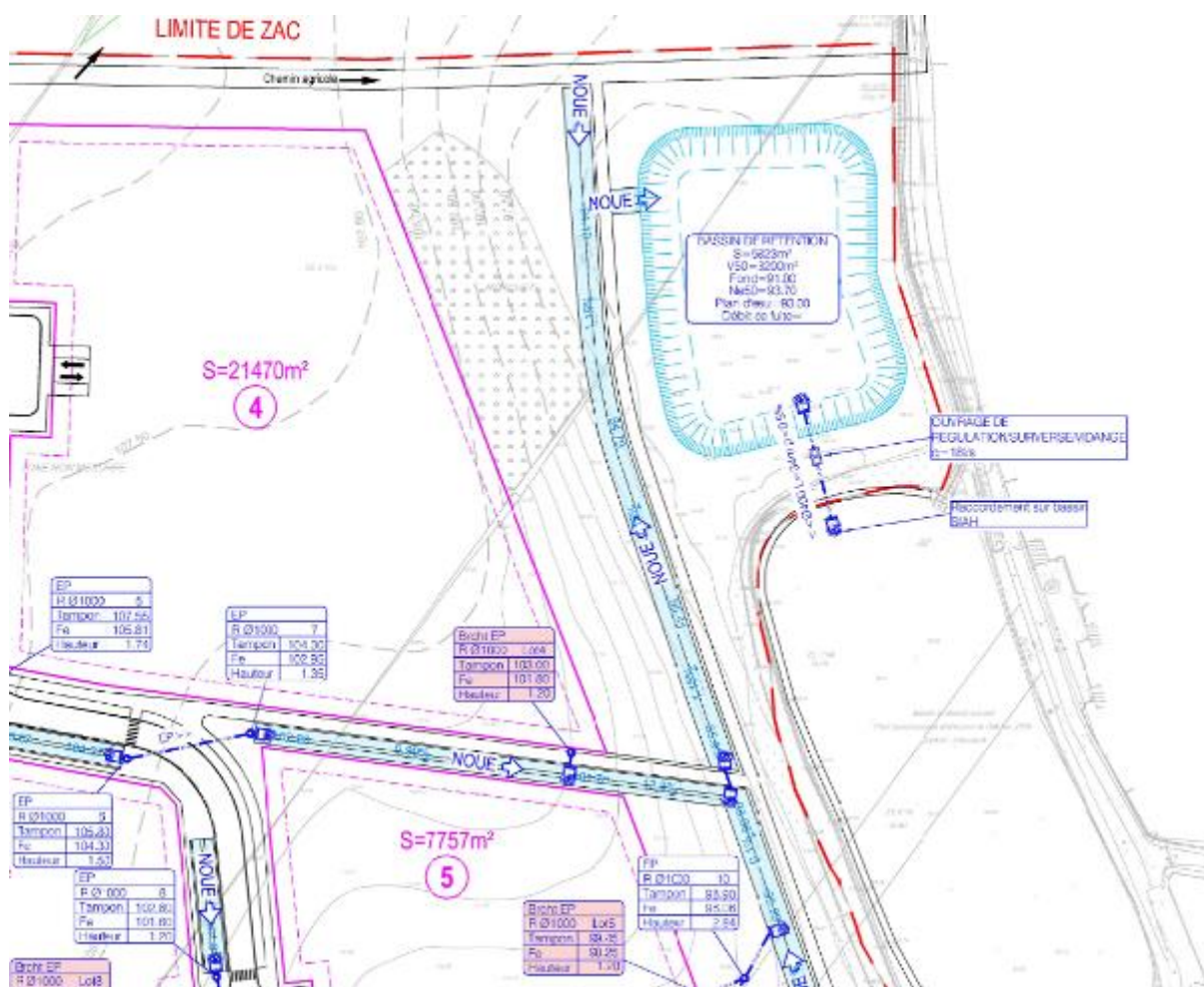
Figure 45 : Fonctionnement du bassin de gestion EP
