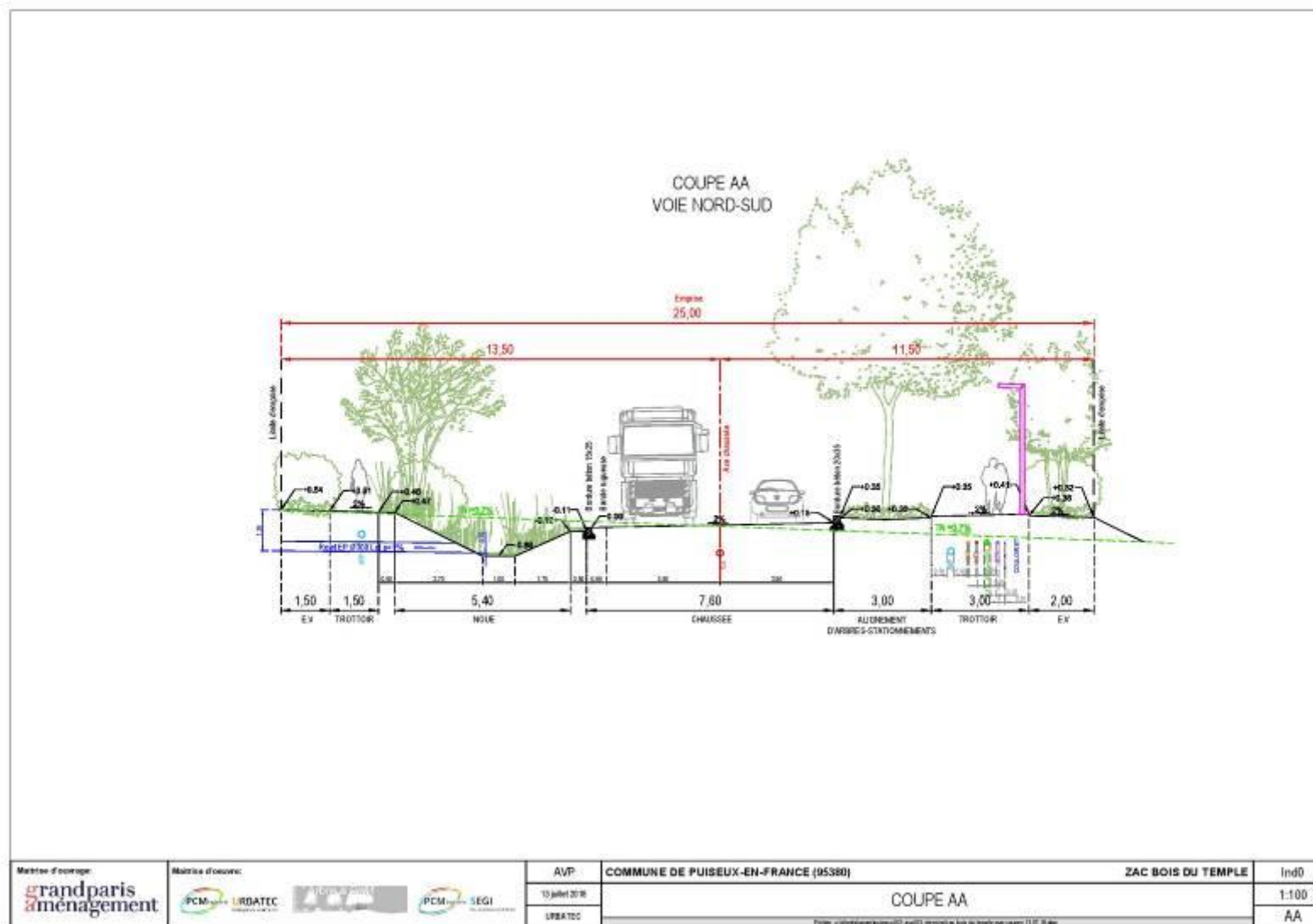
Figure 41 : Coupe de principe sur voirie Nord-Sud
