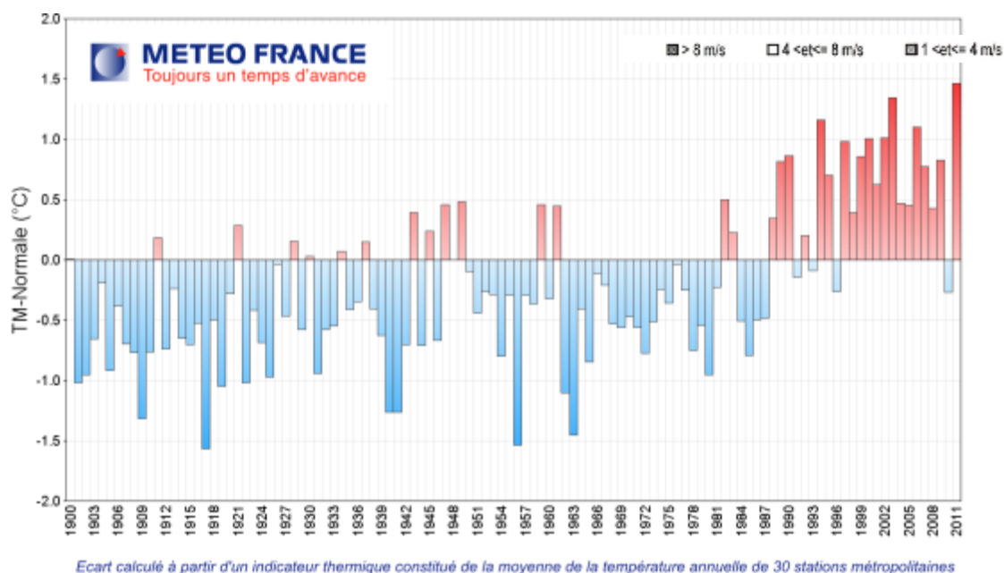
Figure 9 : Evolution de la température annuelle en France
