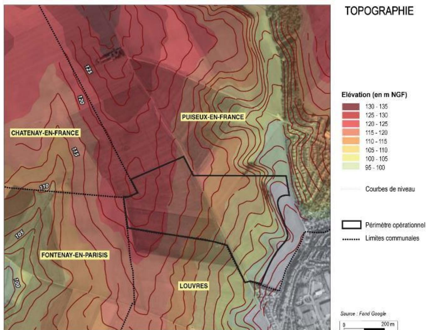
Figure 10 : Carte topographique de la zone d'étude.
