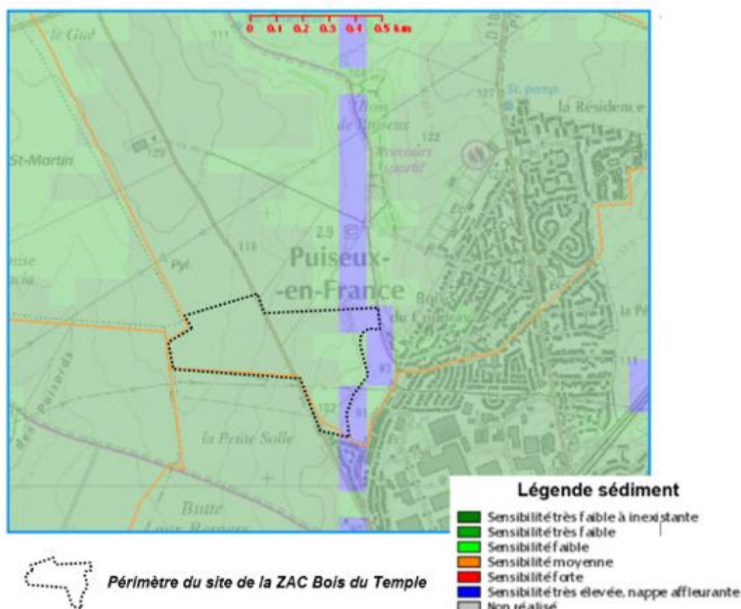
Figure 25 : Détail du zonage de l'aléa « inondation par remontée de nappe »
